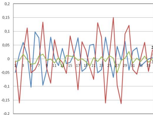
Рис. 4. Смещения по ИТ8 скорости при ближнем очаге.
