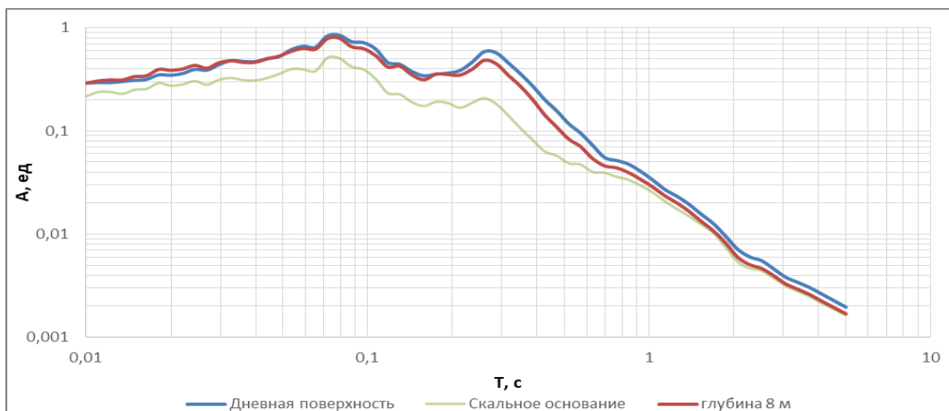
Рис. 6. Спектр реакции грунтовой толщи на различных глубинах.
