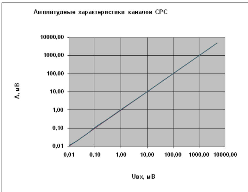
Рис. 10. Амплитудные характеристики каналов СРС сеймостанции Гиссарак ИТ3.
