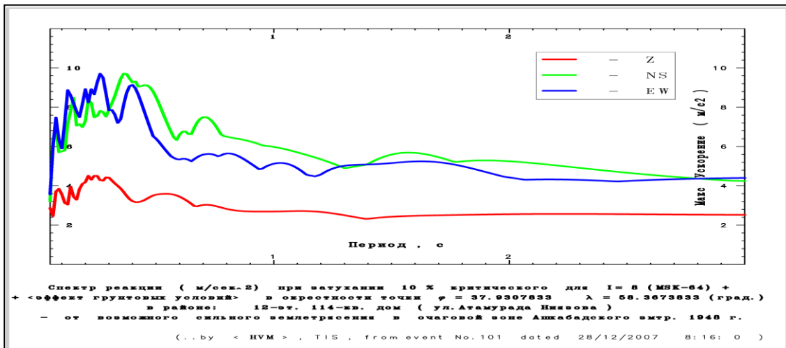
Рис. 9. Спектр реакции одномерного осциллятора с затуханием 10% критического на воздействие ускорений смещений по акселерограмме (см. рис. 8) возможного сильного землетрясения с учетом местных грунтовых условий.
