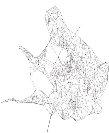
Рис. 2. Дискретизация области СМР треугольниками Делоне (триангуляция Делоне по фактическим точкам наблюдений) на основе соответствующих диаграмм Вороного, вычисляемых методом заметающих плоскостей (S.Fortune, 1987).
