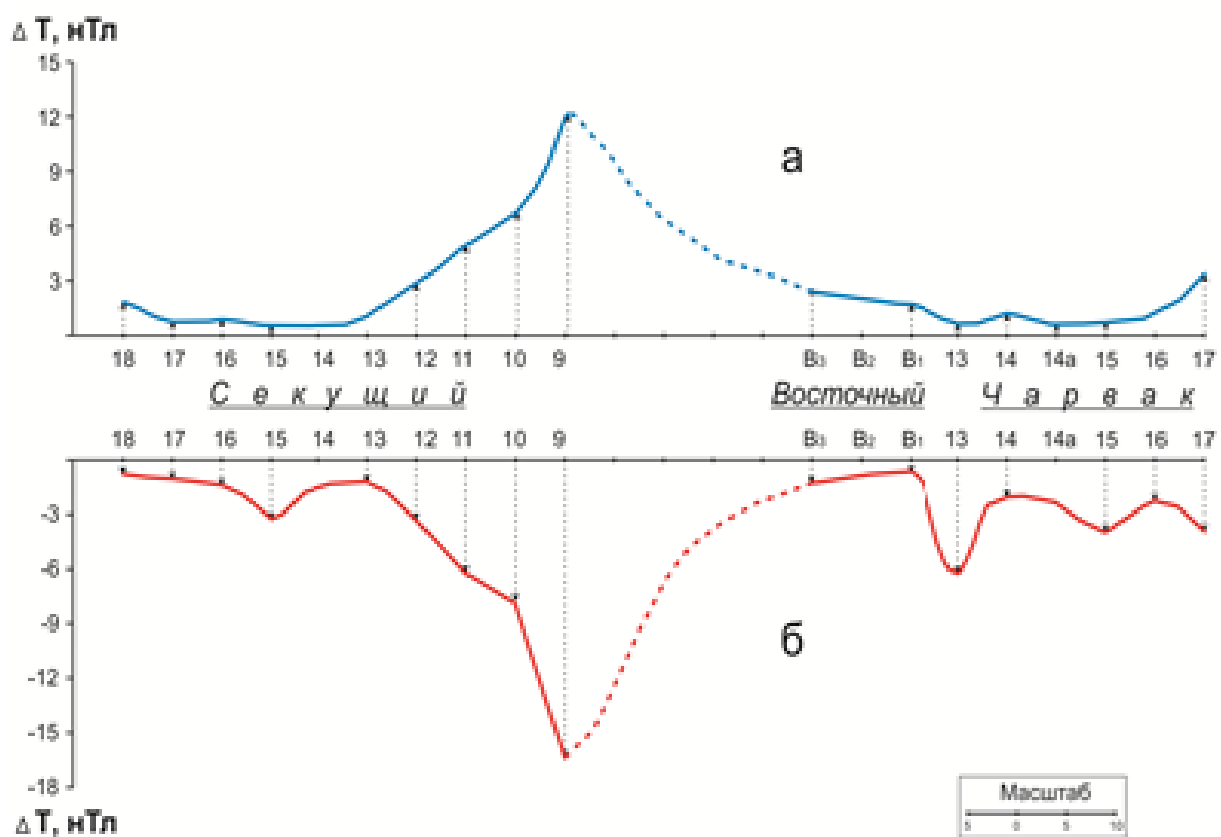
Рис. 3. Аномальные изменения магнитного поля по Секущему и Восточному профилям, связанные с Таваксайским землетрясением 6 декабря 1977 г. M = 5,2 .
