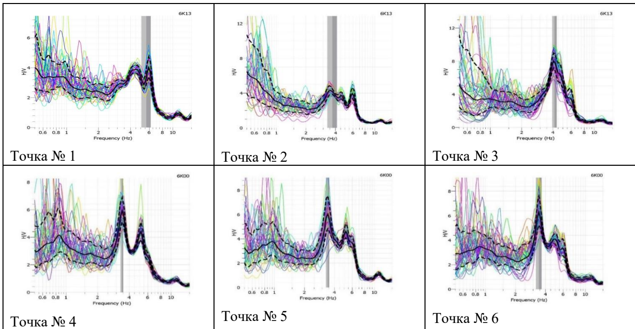
Рис. 7. Спектры HVSr микроколебаний в точках наблюдений.
