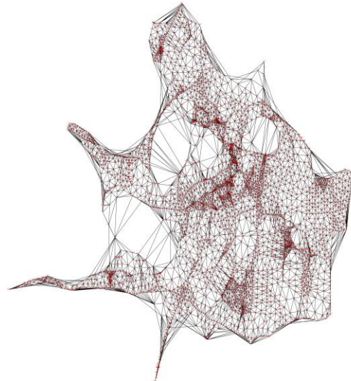
Рис. 3. Дискретизация области СМР треугольниками Делоне (триангуляция Делоне по фактическим точкам наблюдений) на основе соответствующих диаграмм Вороного, вычисляемых методом заметающих плоскостей (S.Fortune, 1987).
