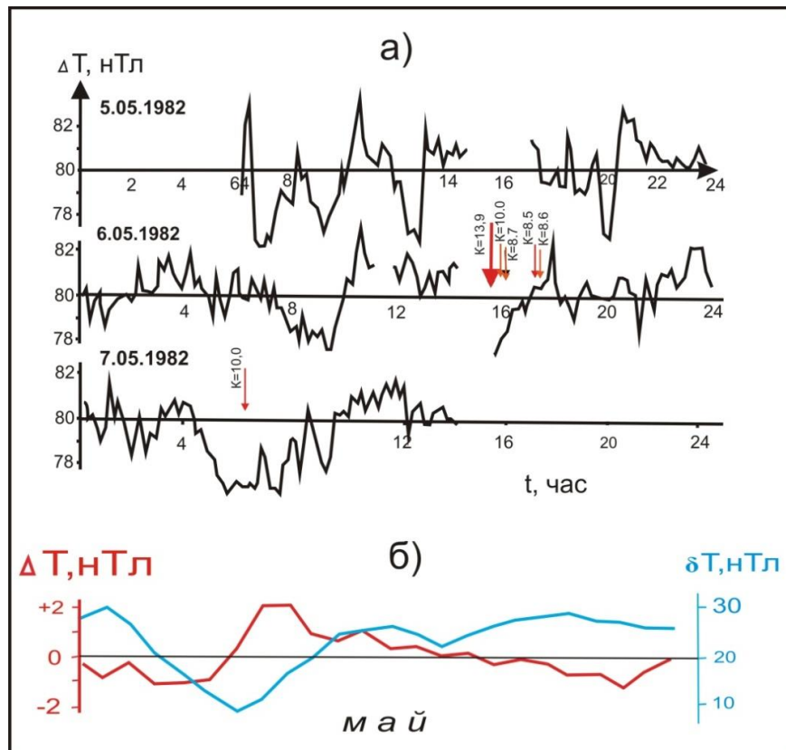
Рис. 2. Вариации магнитного поля над очагом Чимионского землетрясения с M = 5,8 ( K = 13,9 ) до, в момент и после основного толчка и их афтершоков (а) и средненормированные ходы за май 1982 г. среднесуточного наблюдаемого хода \delta T и среднесуточных разностей \Delta T между ст. Чимион и обсерваторией Янгибазар (б).
