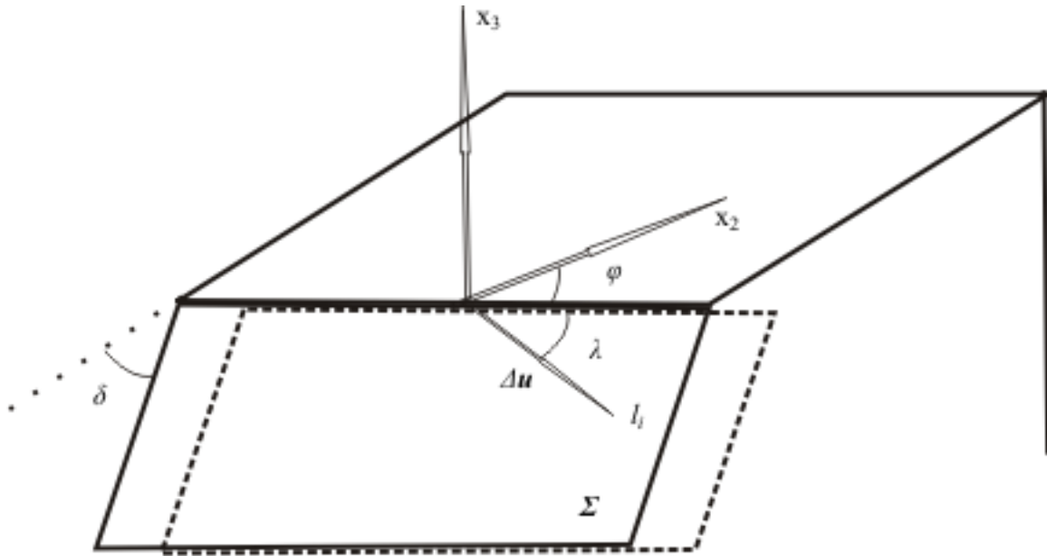
Рис. 1. Плоскость разрыва при землетрясении.
