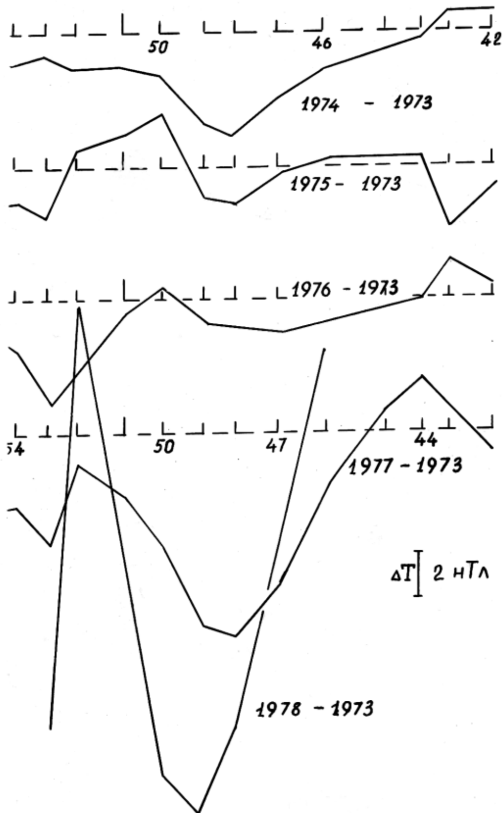
Рис. 4. Аномальные изменения магнитного поля по профилю Маданият-Карасу, связанные с Алайским землетрясением 1 ноября 1978 г. (M = 6,8).
