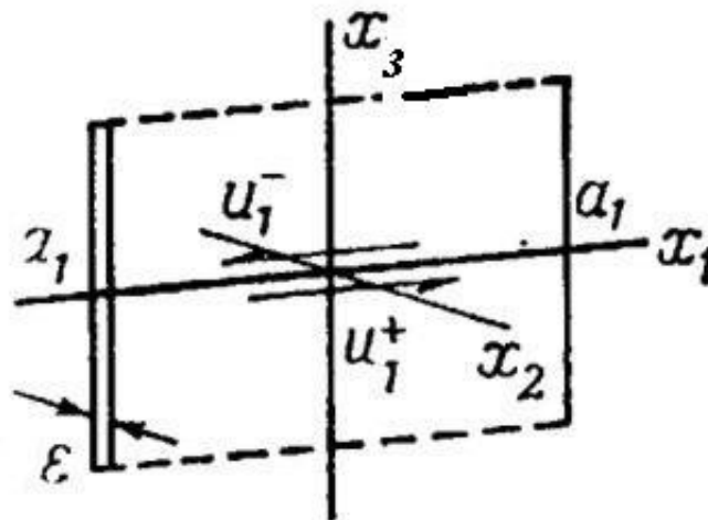
Рис. 3. Пример получения эквивалентных сил при дислокации вдоль оси x_1 .
