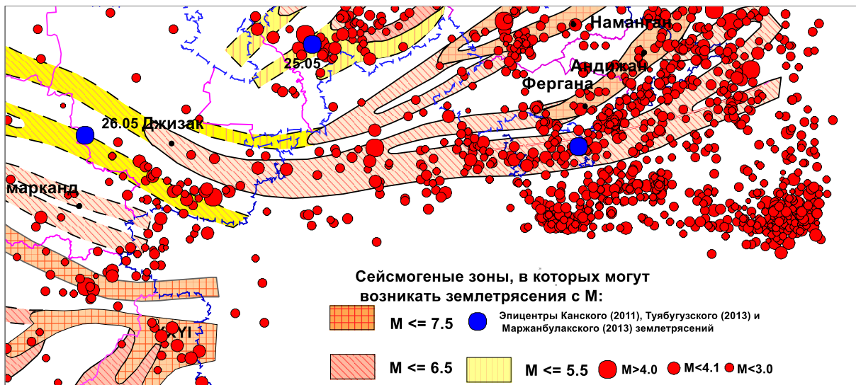
Рис. 3. Пространственное распределение слабых землетрясений за 2016-2017 гг. (по данным РЦСМ МЧС РУз.).
