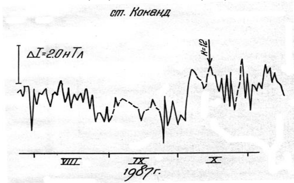
Рис. 15. Ступенчатая специфическая аномалия на ст. Коканд перед землетрясением 14.10.1987 г. с K = 12 .
