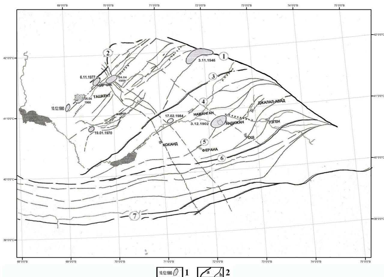
Рис. 2. Активные разломы и изосейсты сильных землетрясений Западного Тянь-Шаня. 1 – изосейсты землетрясений; 2 – активные разломы земной коры: а – краевые: 1 – Таласо-Ферганский, 2 – Аксу-Майдантальско-Богоналинский, 3 – Северо-Ферганский, 4 – Северо-Ферганская ФРЗ, 5 – Южно-Ферганская ФРЗ, 6 – Южно Ферганский, 7 – Гиссаро-Кокшаальский; б – внутренние.
