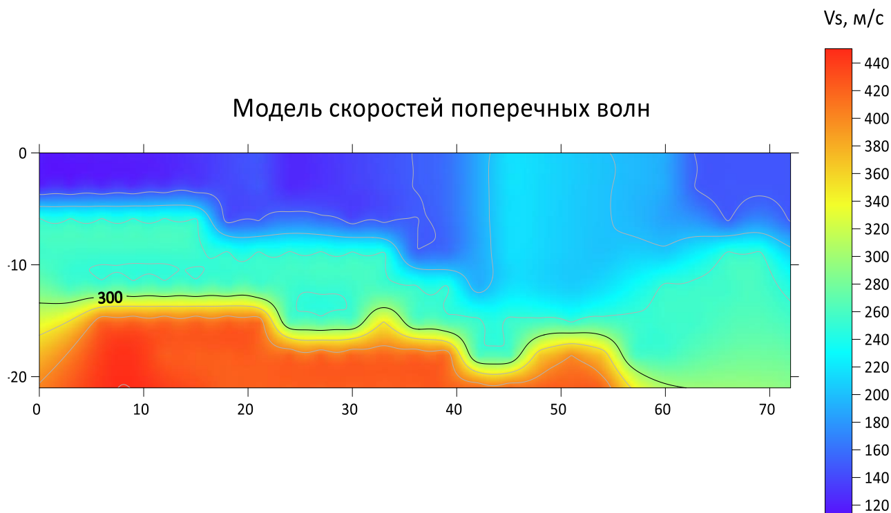
Рис. 3. Скоростной ( V_s ) разрез грунтовых толщ на площади расположения многоэтажного жилого дома.
