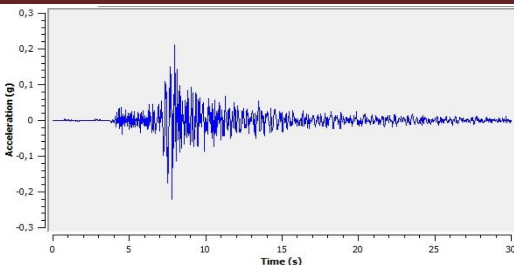
Рис. 4. Нормализованная акселерограмма землетрясения Таш-Добо, Киргизия. Запись станции СНМАЕ 26.12.2020 г.
