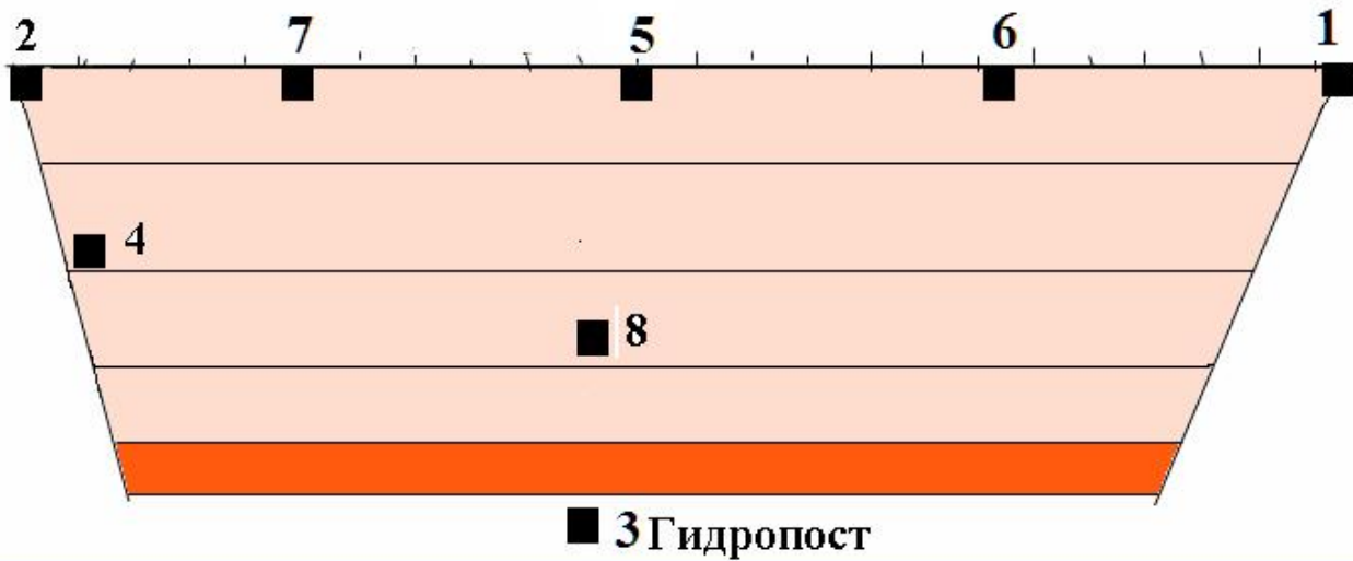
Рис. 1. Схема размещения измерительных точек на плотине в береговых склонах Гиссарского водохранилища.
