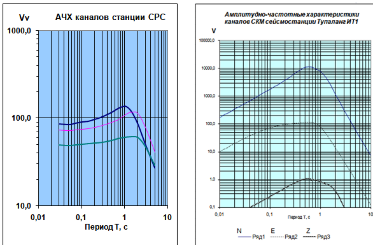
Рис. 11. АЧХ характеристики каналов СКМ сеймостанций Тупаланг ИТ1.
