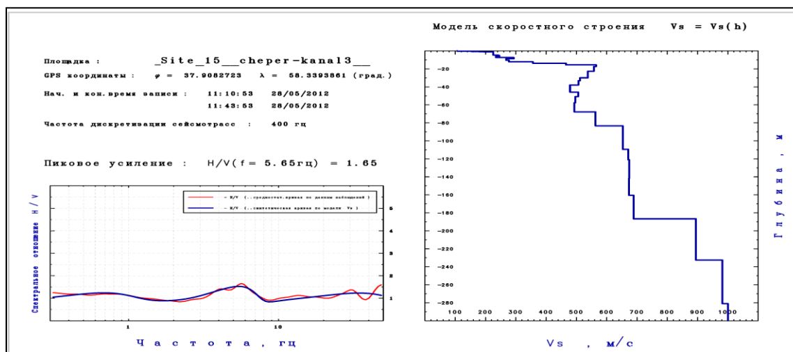
Рис. 5. Многослойная модель второго уровня детальности на основе скоростной модели первого уровня детальности (см. рис. 1) в том же пункте обследования с использованием данных по соседним точкам.
