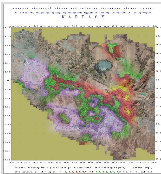
Рис. 11. Предварительная карта приращений балльности по локальным грунтовым условиям относительно эталонной площадки в районе Министерства образования.
