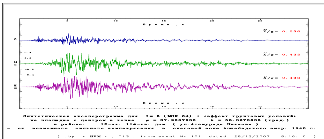
Рис. 8. Пример пересчета записи слабого землетрясения в акселерограмму возможного сильного землетрясения с учетом местных грунтовых условий.
