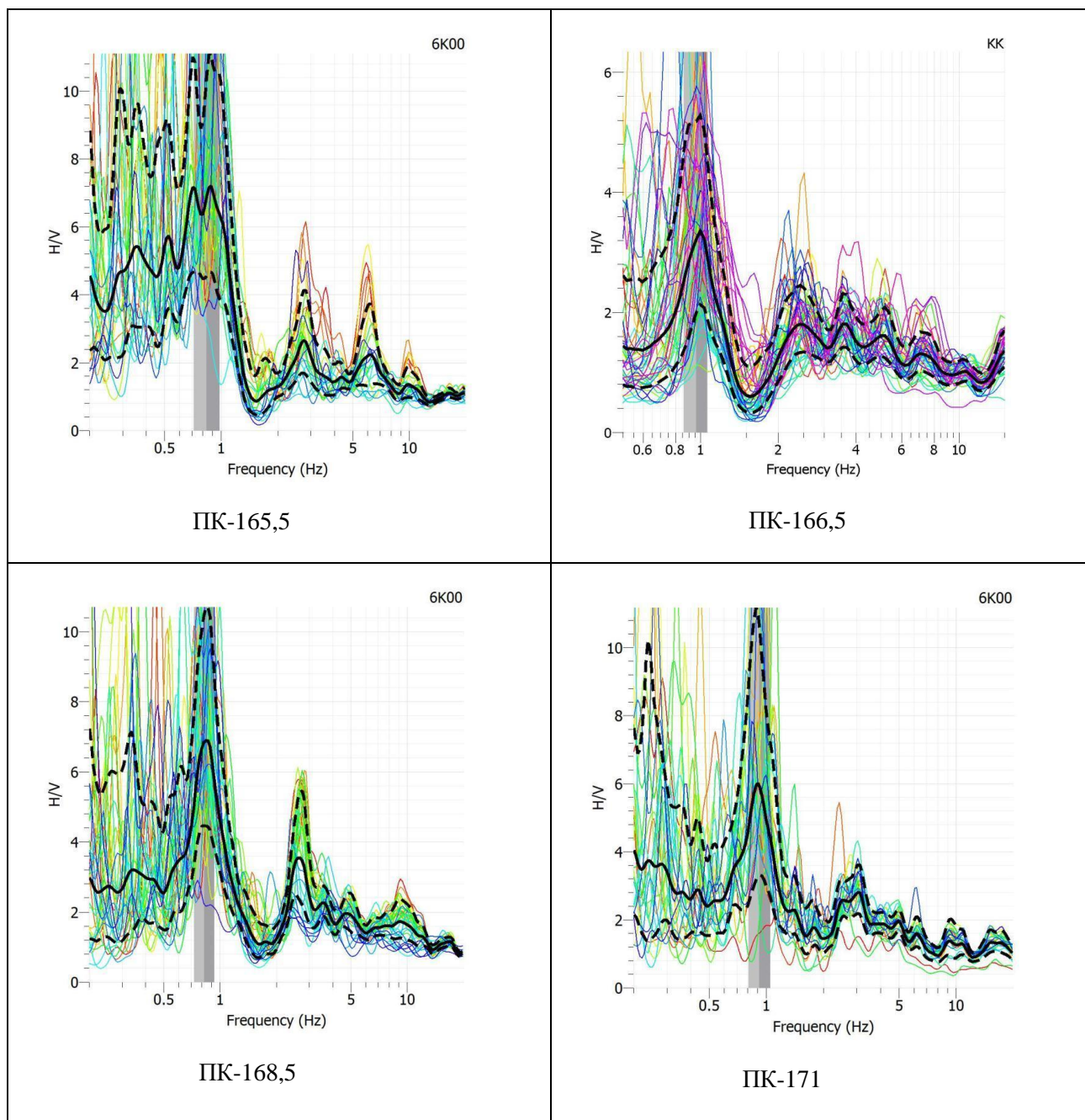
Рис. 3. Спектры HVSR, полученные для пунктов регистрации № 165,5; 166,5; 168,5; 171.
