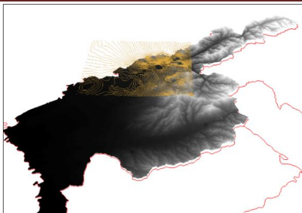
6-расм. Чорвоқ сув омбори ҳудудининг RBM рақамли баландлик модели.
