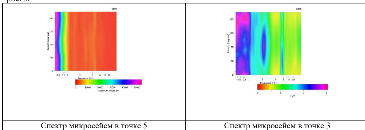
Рис. 3. Спектры микросейсм в точках 3 и 5.
