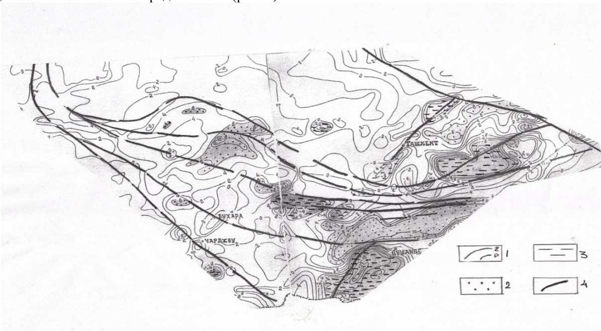
Рис. 4. Фрагмент схематической карты современных движений Земной коры Средней Азии [14], с добавлениями (активные разломы). Масштаб 1: 2 500 000. 1 – изолинии скоростей вертикальных движений, мм / год; 2, 3 – участки поднятий и опусканий; 4 – разрывные нарушения, новейшая и современная активность которых доказана данными сейсмичности.
