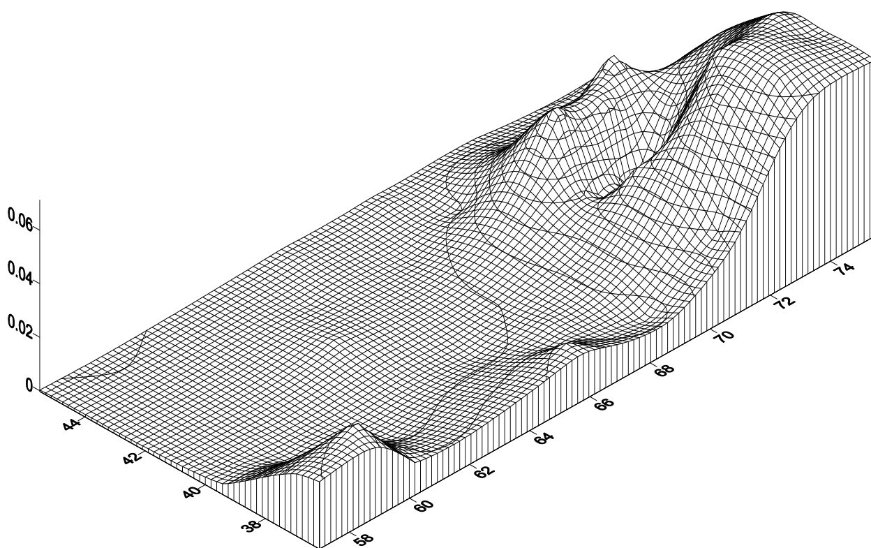
Рис. 7. Один из вариантов окончательного рельефа после проведения численного эксперимента с использованием реального рельефа, приведенного на рис. 2. По горизонтали – восточная долгота и северная широта в градусах. По вертикали – высота в масштабе 1:100 км.
