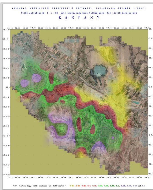
Рис. 12. Предварительная карта значений параметра Vs30 по результатам HVSR-анализа данных микросейсмического обследования.
