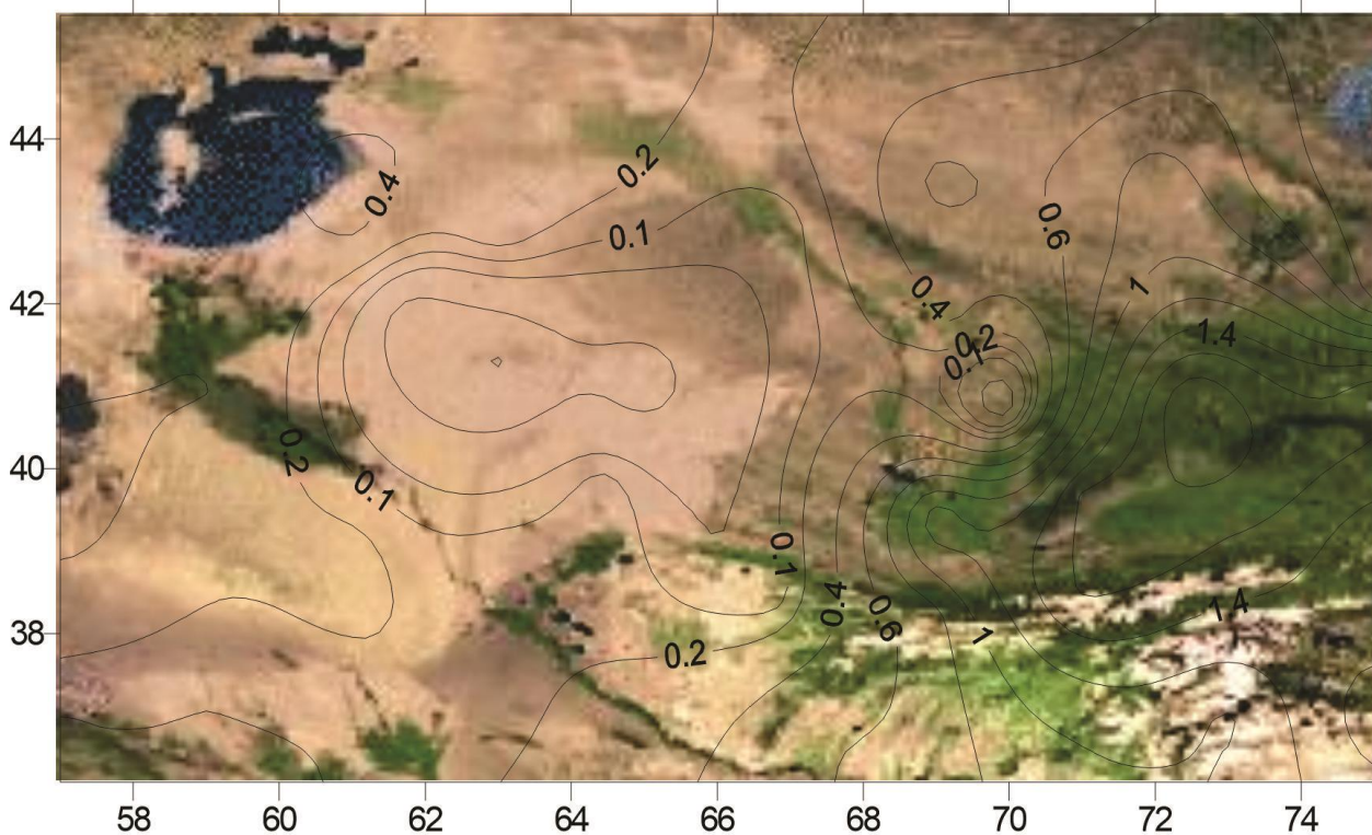
Рис. 8. Интенсивность касательных напряжений (в 10^2 МПа) на глубине 20 км, полученная при решении обратной задачи.
