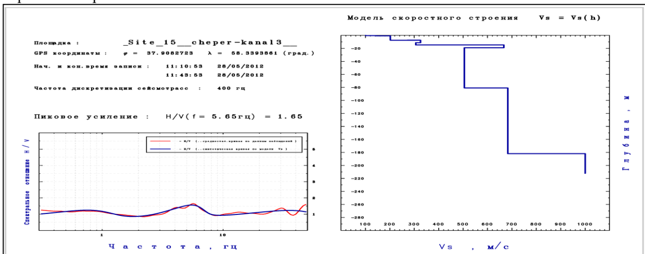
Рис. 1. Пример модели первого уровня детальности для одной из обследованных площадок.
