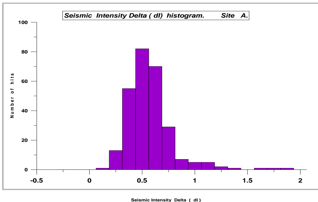
Рис. 10. Гистограмма приращений сейсмической балльности \Delta I (MSK-64) для одной из точек обследования по акселерограммам возможных сильных землетрясений.
